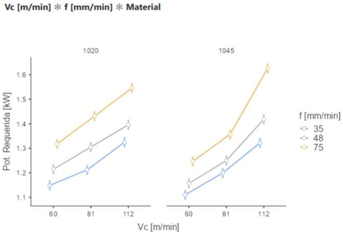
Figura 33 - Estimativa Marginal Média para os valores da Potência Requerida
