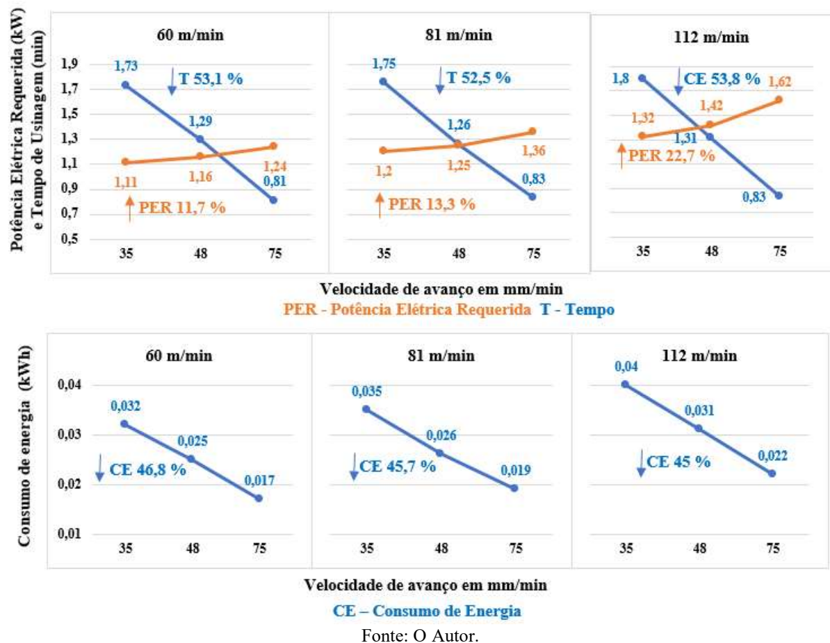
Figura 25- Potência elétrica requerida, tempo de usinagem e consumo de energia no aço ABNT 1045.
