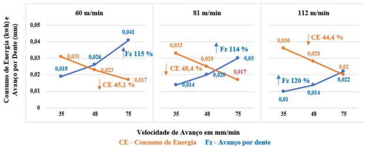
Figura 19 - Consumo de energia e avanço por dente no aço ABNT 1020.
