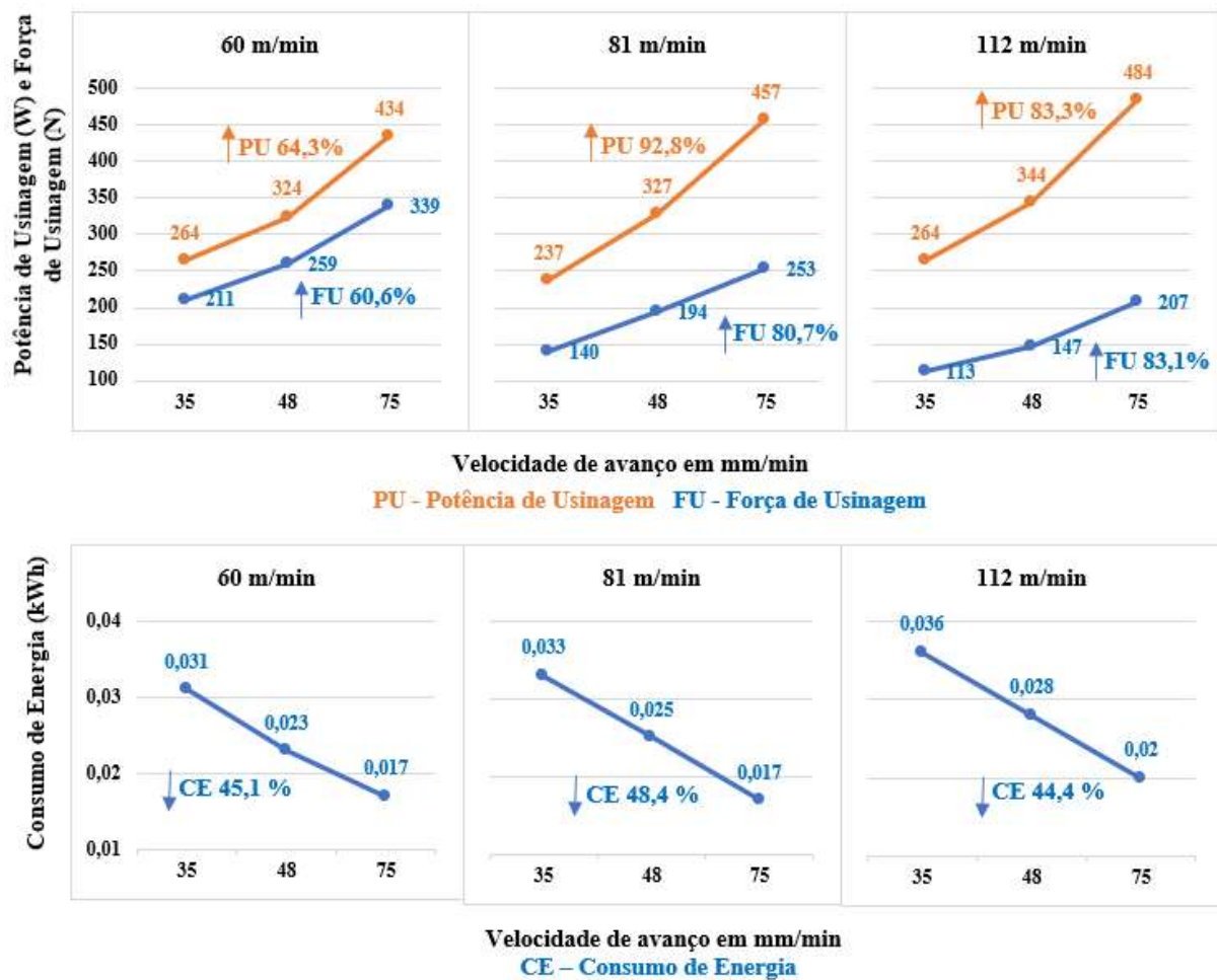
Figura 22 - Força de usinagem, potência de usinagem e consumo de energia em função da velocidade de avanço no aço ABNT 1020.
