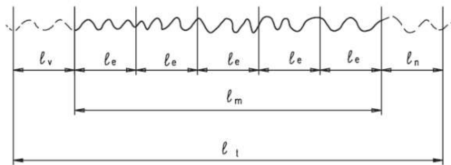
Figura 7 - Comprimentos para a avaliação da rugosidade.
