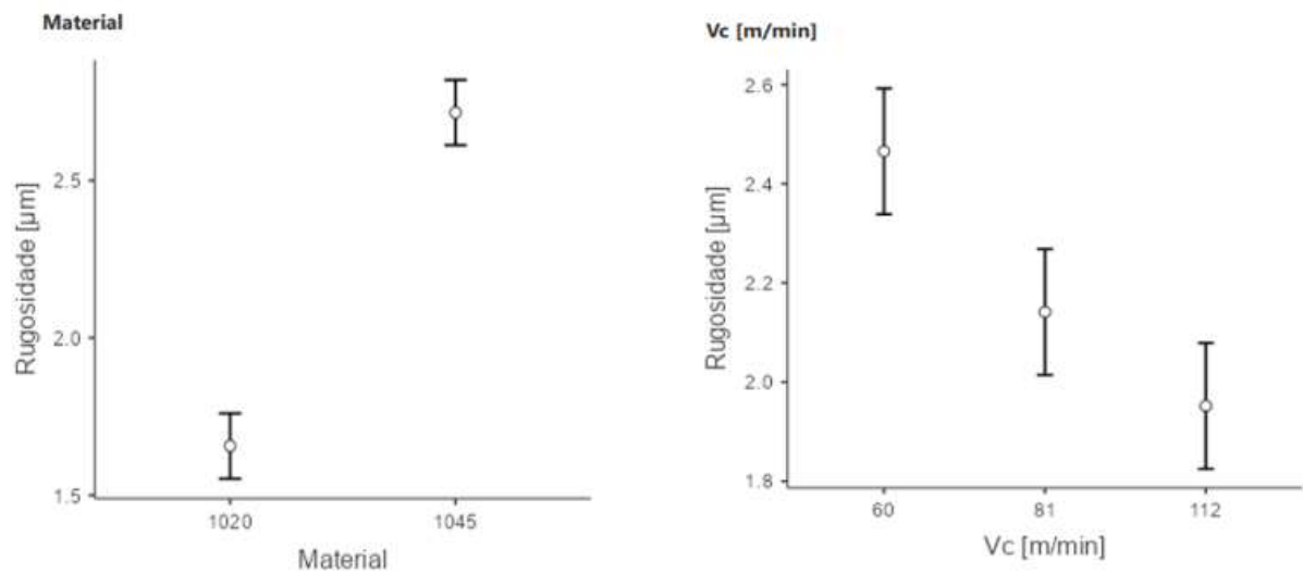
Figura 29- Estimativa Marginal Média para os valores de Rugosidade
