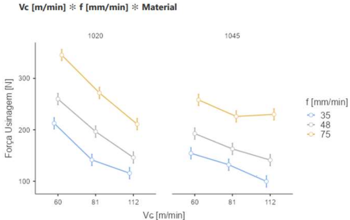
Figura 31 - Estimativa Marginal Média para os Valores de Força de Usinagem
