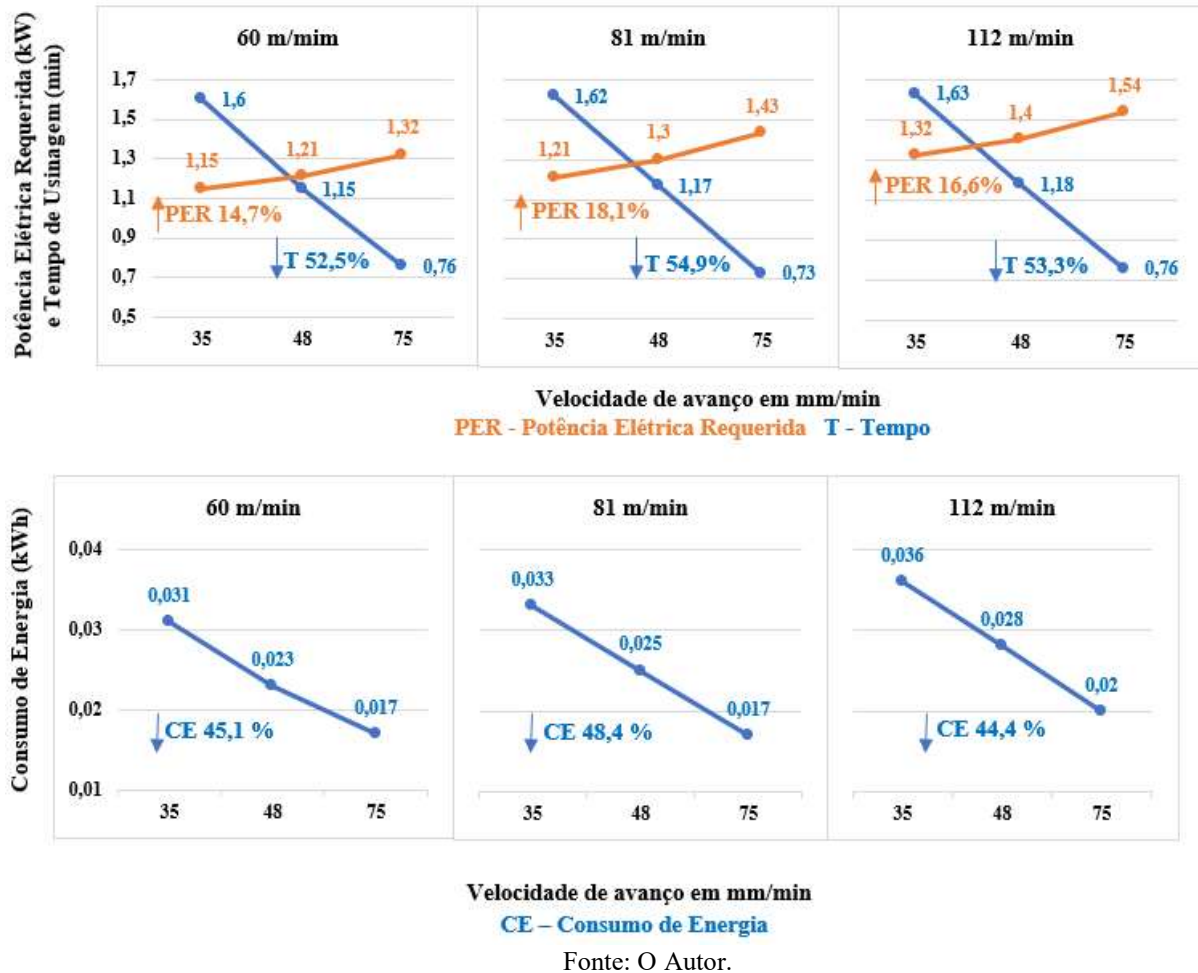
Figura 20 - Potência elétrica requerida, tempo de usinagem e consumo de energia no aço ABNT 1020.
