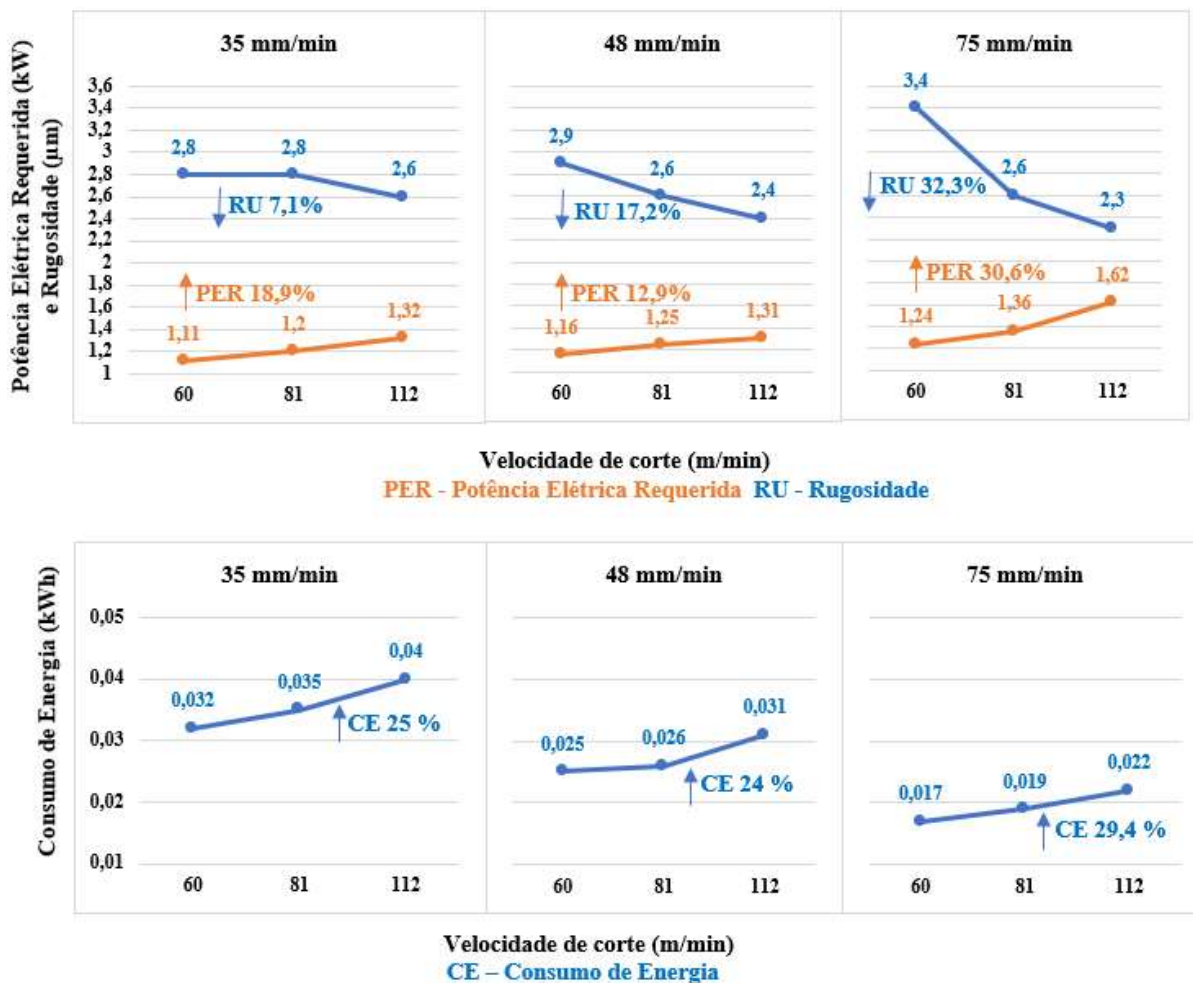
Figura 23 - Rugosidade Final, Potência elétrica requerida e consumo de energia no aço ABNT 1045.
