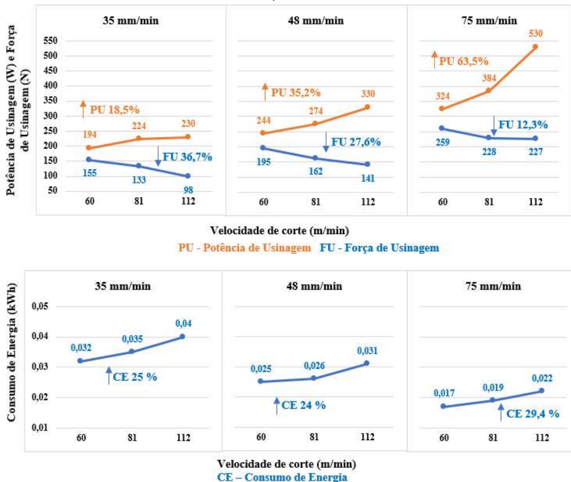
Figura 26 - Força de usinagem, potência de usinagem e consumo de energia em função da velocidade de corte no aço ABNT 1045.
