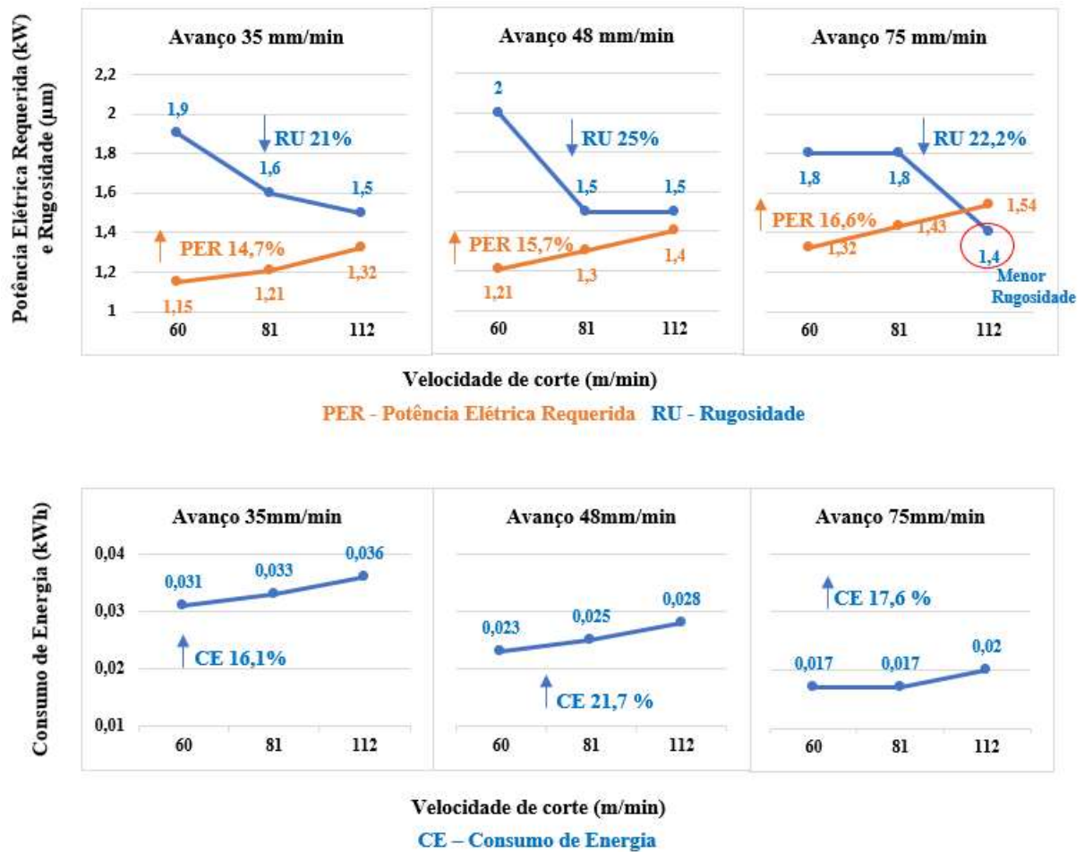
Figura 18 - Rugosidade Final, Potência elétrica requerida e consumo de energia no aço ABNT 1020.
