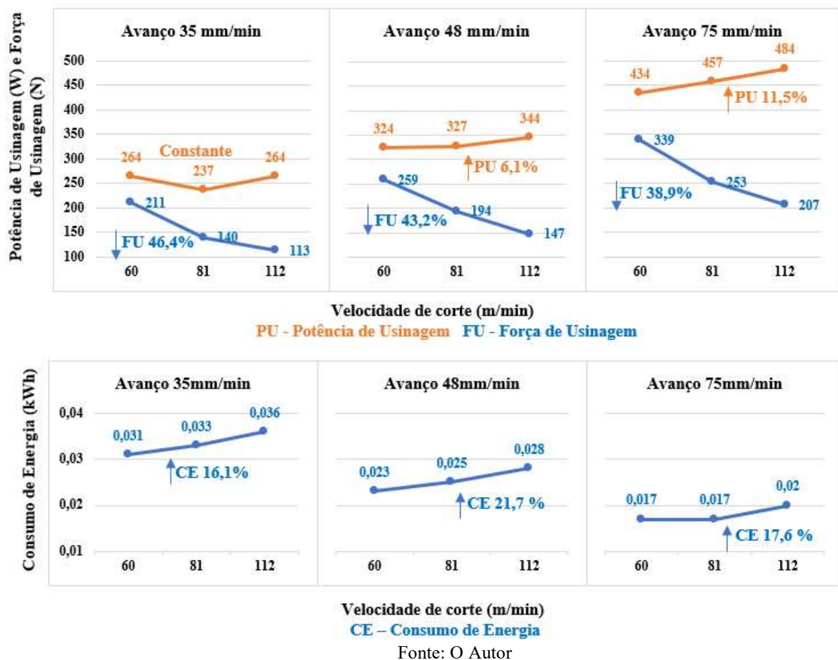
Figura 21 - Força de usinagem, potência de usinagem e consumo de energia em função da velocidade de corte no aço ABNT 1020.
