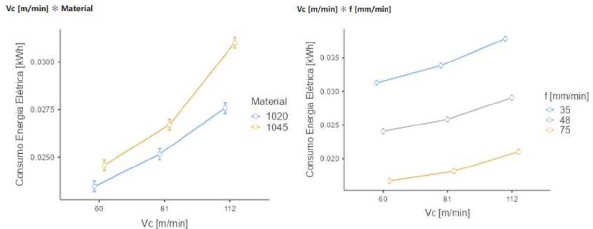
Figura 35 - Estimativa Marginal Média para os valores do Consumo de Energia
