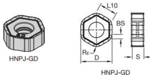
Figura 11 - Dimensões do inserto.
