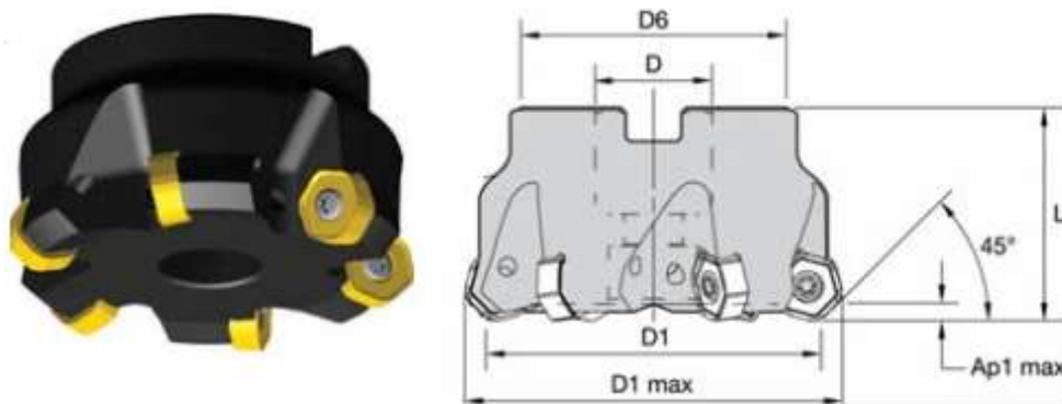
Figura 10 - Cabeçote fresador.
