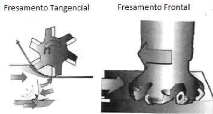
Figura 3 – Tipos de Fresamentos.
