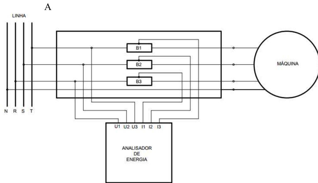
Figura 15 - Bancada Teste - a) Esquema elétrico, b) Modelo real.
