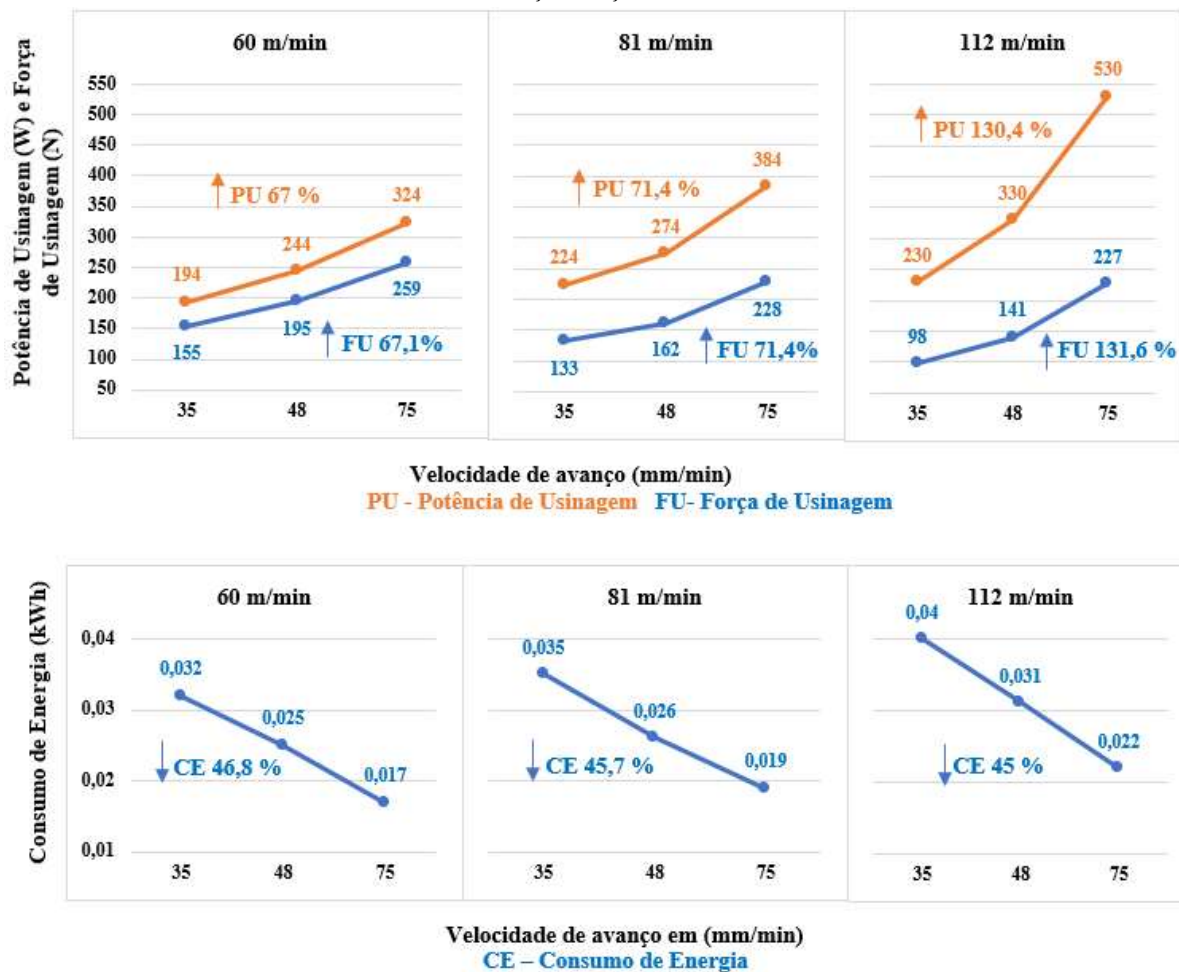
Figura 27 - Força de usinagem, potência de usinagem e consumo de energia em função da velocidade de avanço no aço ABNT 1045
