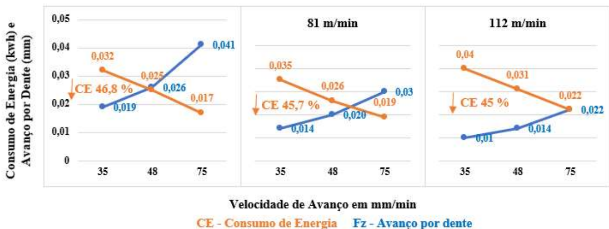
Figura 24 - Consumo de energia e avanço por dente no aço ABNT 1045.
