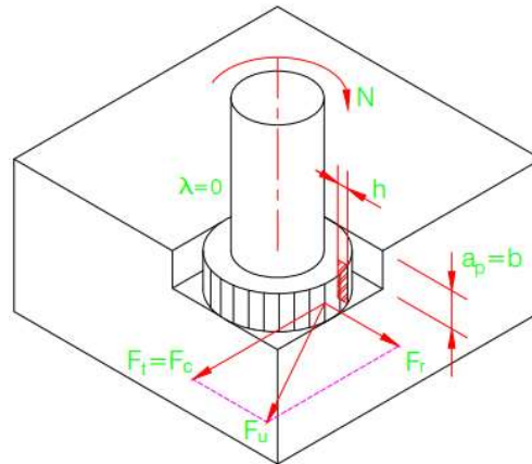
Figura 4 - Componentes da força de usinagem no fresamento frontal.
