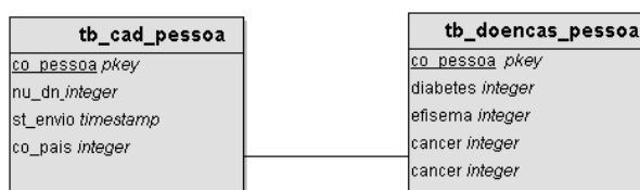
Figura 16 – Exemplo de tabela em relacional.
