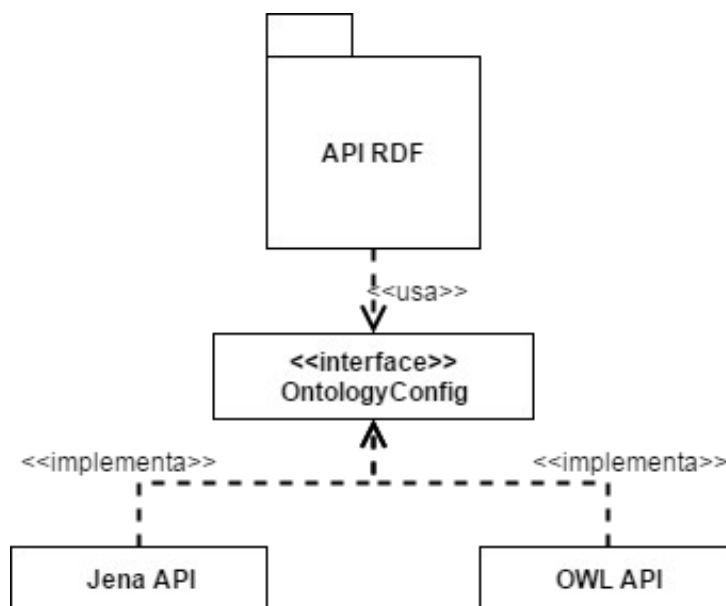
Figura 31 – Exemplo de independência de API
