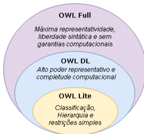
Figura 8 – Representatividade das sub-linguagens de OWL como Diagramas de Venn
