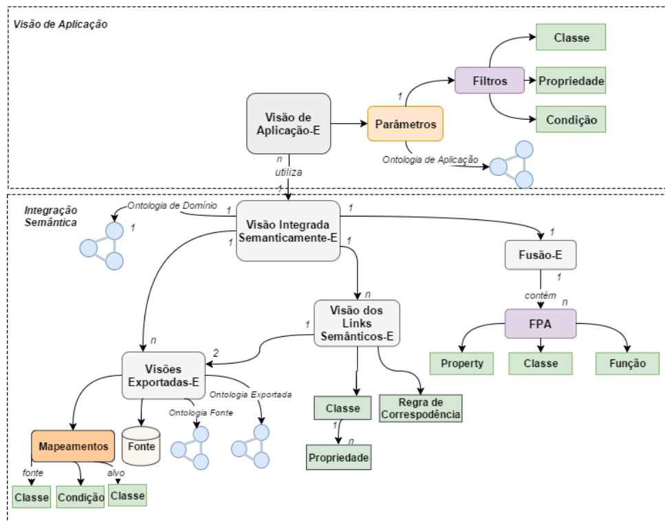
Figura 30 – Modelo Conceitual Mediador Semântico
