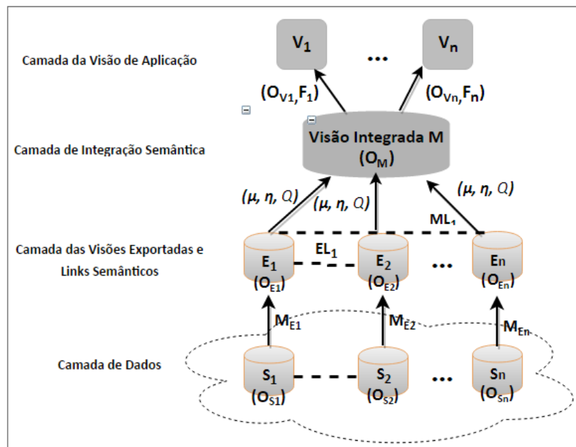
Figura 29 – Arquitetura 4 Camadas do Mediador Semântico
