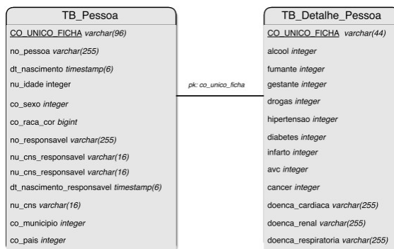
Figura 25 – Visão da base de dados e-SUS
