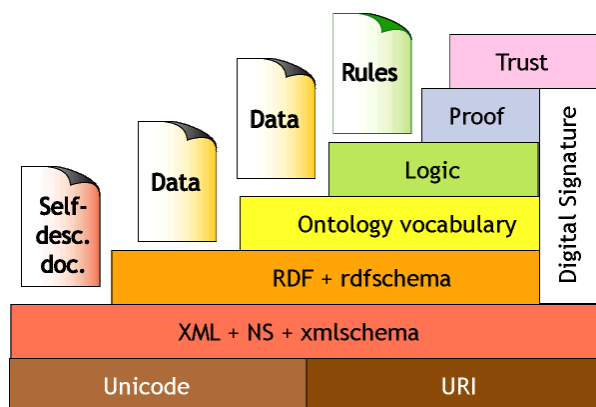
Figura 3 – Camadas da Web Semântica
