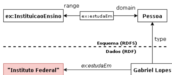
Figura 6 – Exemplo de inconsistência perceptível ao OWL
