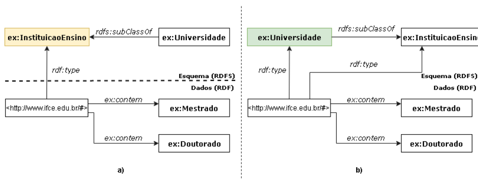
Figura 7 – Exemplo de ação do raciocinador
