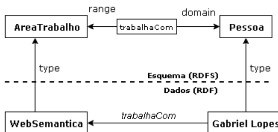
Figura 5 – Relacionamento de RDF e RDFS
