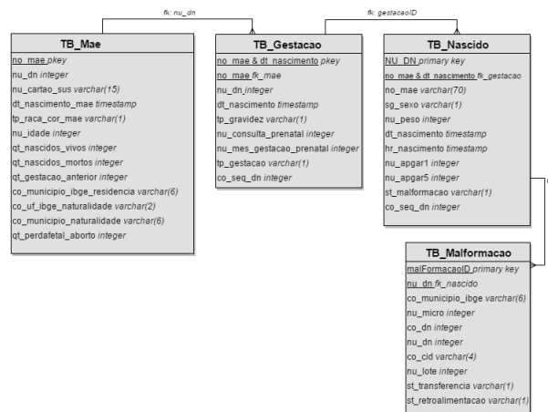
Figura 24 – Visão da base de dados SINASC
