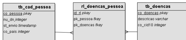
Figura 17 – Outra possibilidade de representação.
