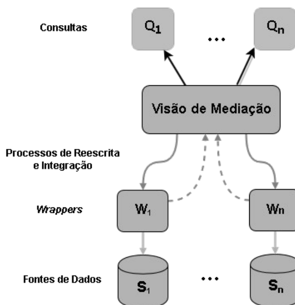
Figura 13 – Arquitetura de um mediador genérico.
