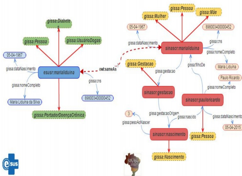
Figura 27 – Instâncias das Visões Exportadas
