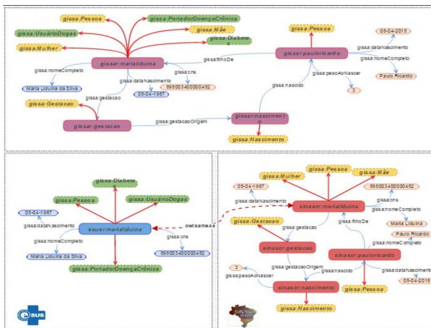
Figura 28 – Instâncias da Visão de Mashup materializada
