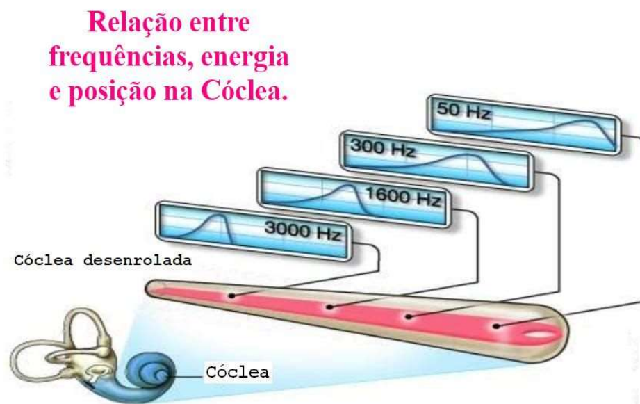
Figura 19: Funcionamento da Cóclea humana
