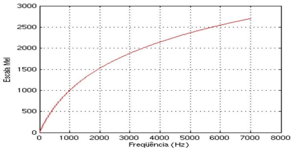
Figura 11: Relação entre a escala Hz e escala mel
